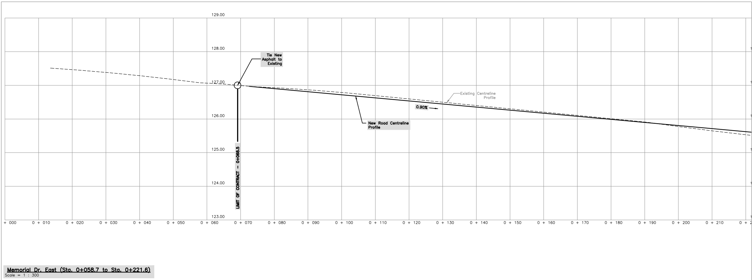
Memorial Dr. East (Sta. 0+058.7 to Sta. 0+221.6) Scale = 1 : 300
